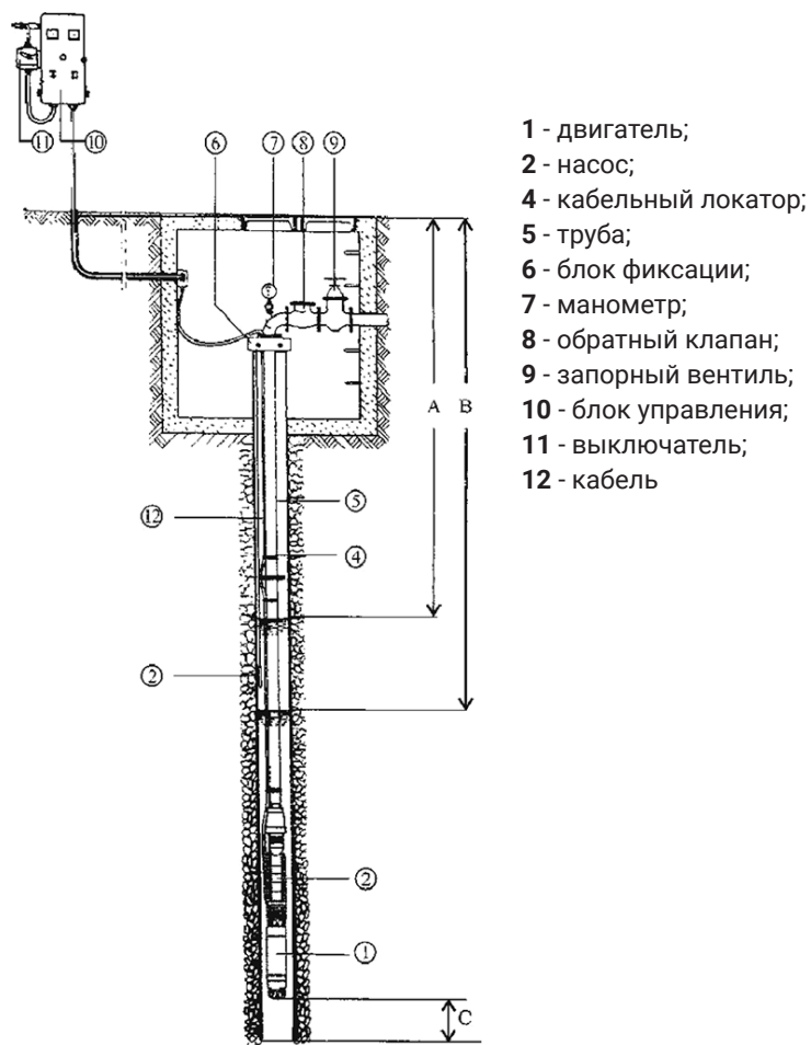
Схема подключения насоса
